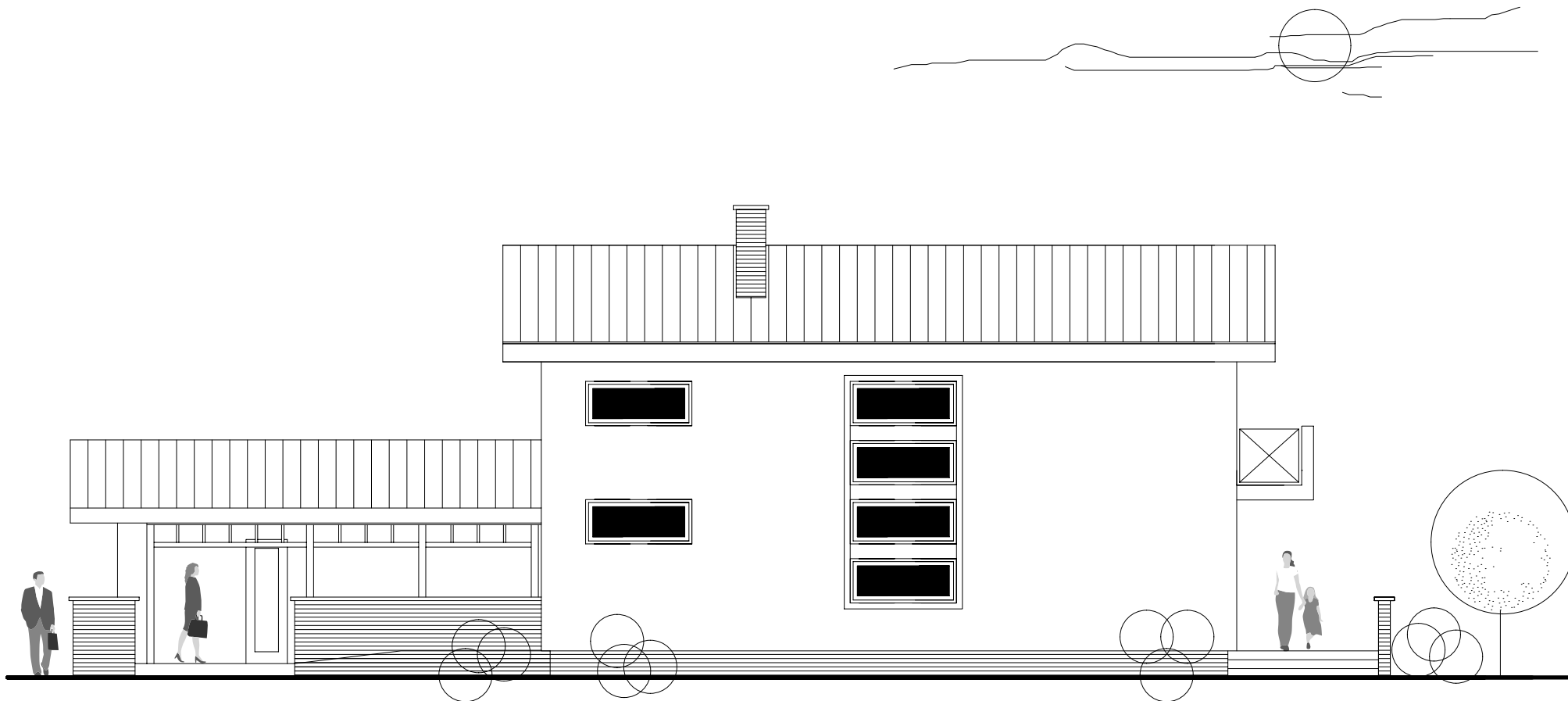
Pohľad západný
